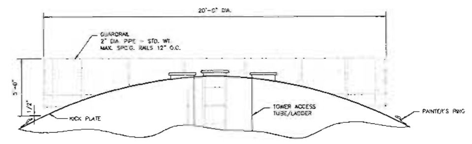
2 SECTION -- TANK GUARDRAIL SCALE: NONE
