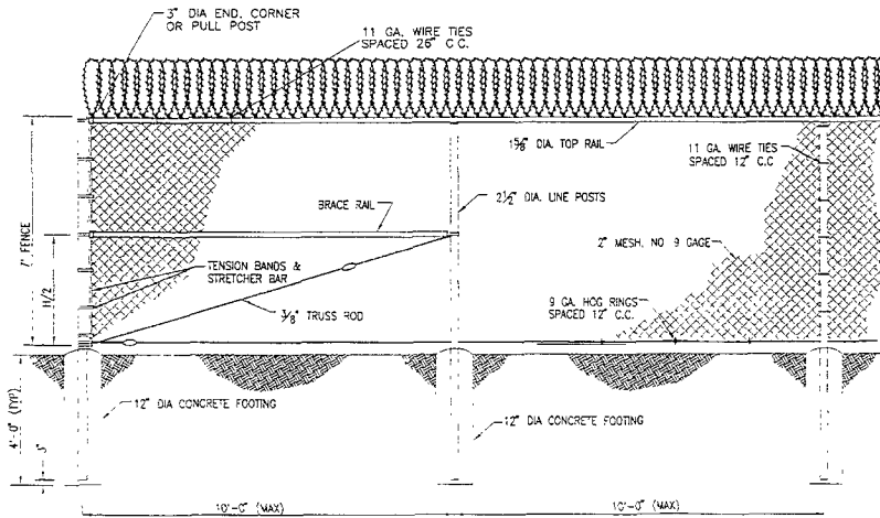
CHAIN LINK FENCE N.T.S.
