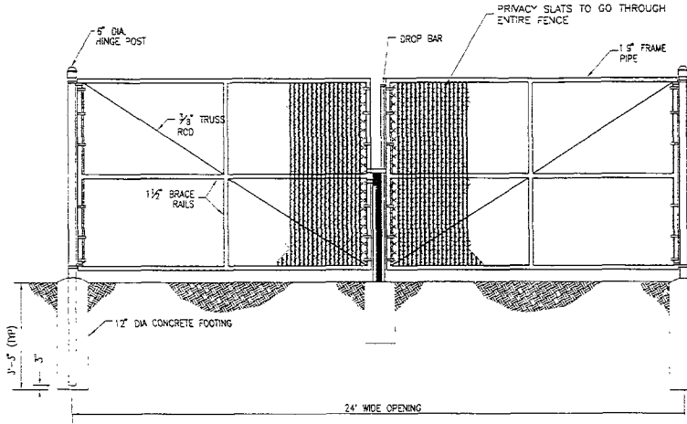
CHAIN LINK FENCE GATE N.T.S.
