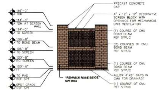
3 ELEVATION
