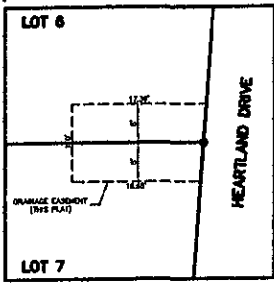
DETAIL SCALE: 1" = 10'
