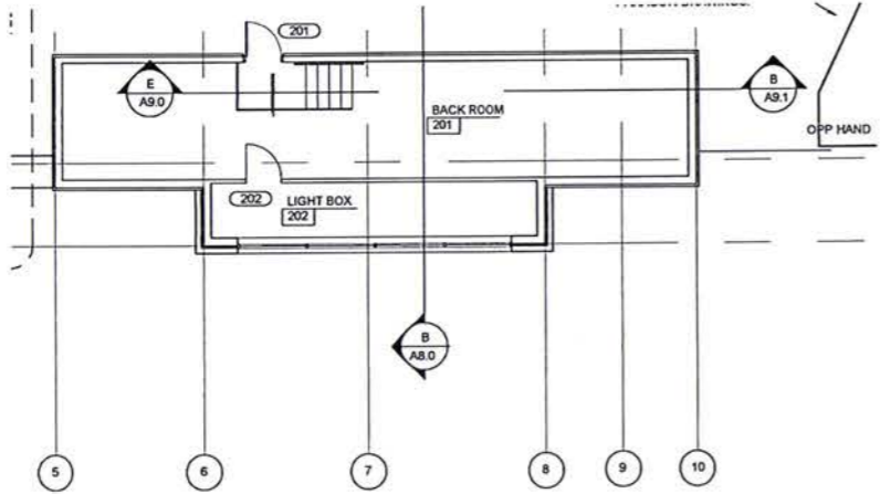
B FLOOR PLAN SCALE: 1/8" = 1'-0"
