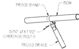
DETAIL - B SCALE: 1/2\"/>
