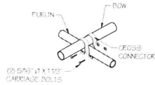
DETAIL - A SCALE: 1/2\"/>
