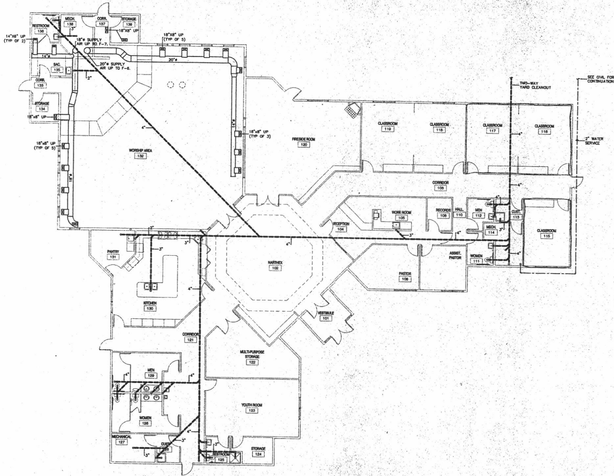
M2 BELOW GRADE PLAN SCALE: 1/8" = 1'-0"
