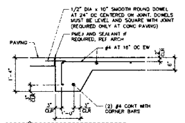
11 NEW SLAB SCALE: 3/4" = 1'-0"
