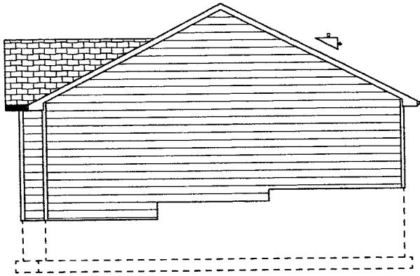
RIGHT ELEVATION
