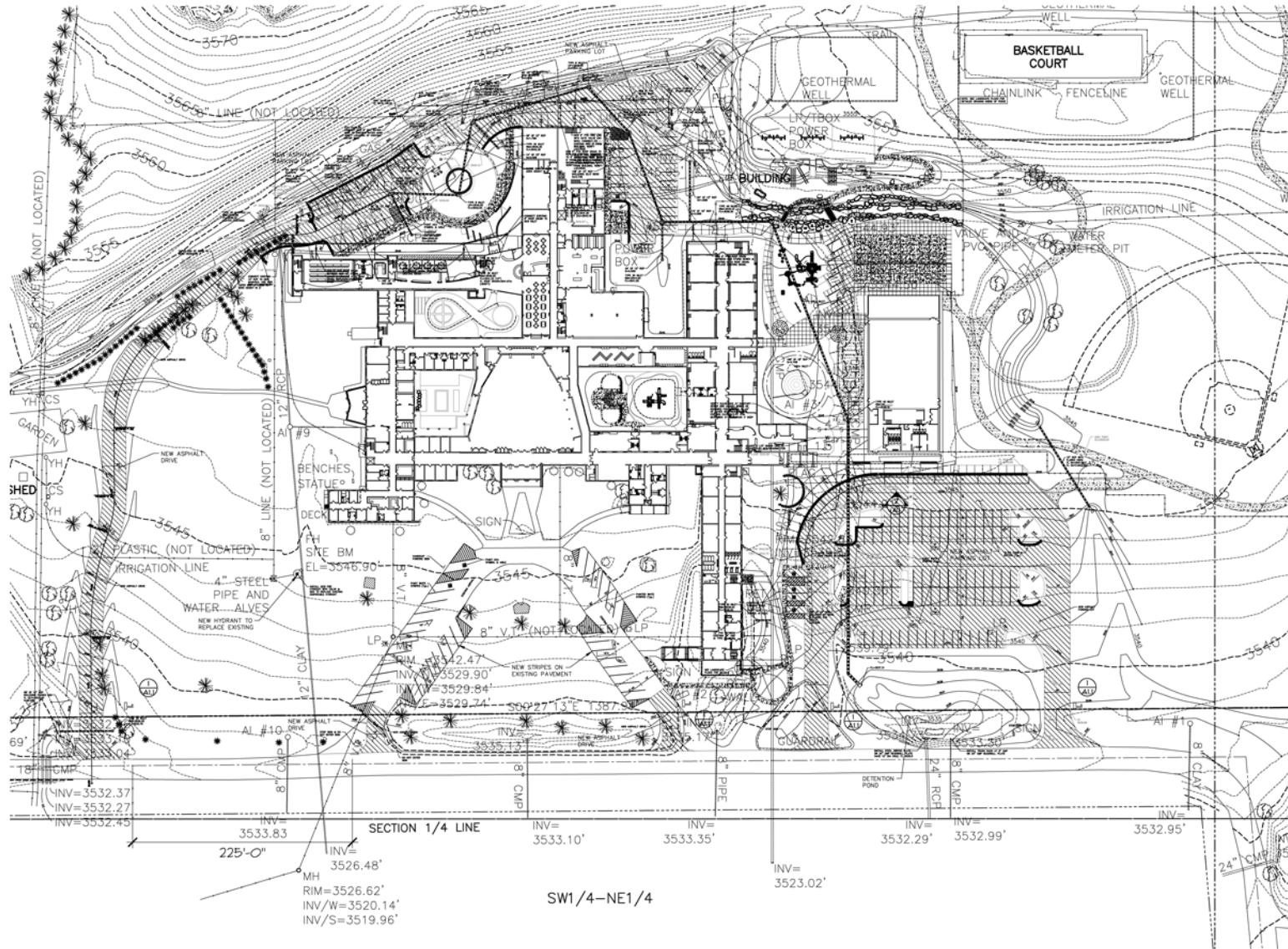
SITE PLAN NT5
