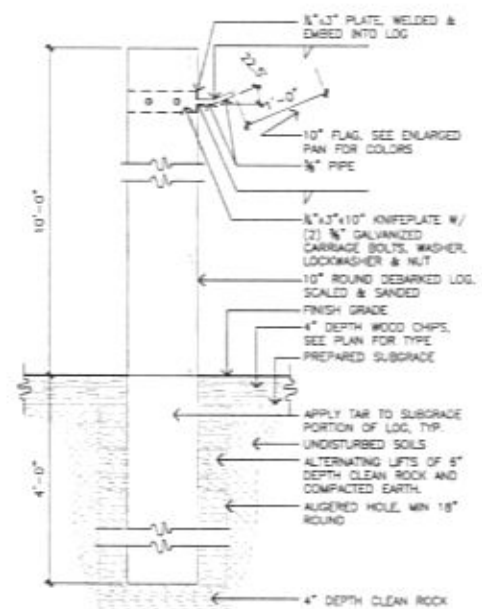
2 DETAIL: TOTEM POLE L2.25 SCALE: 1" = 1'-0"
