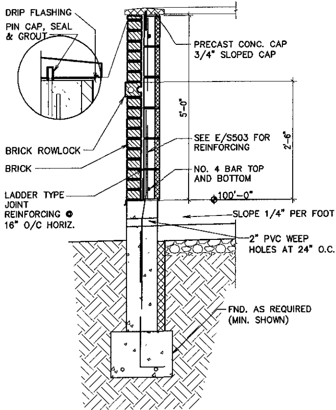
(A) WALL DETAIL N.T.S.
