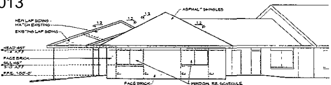
2 WEST ELEVATION 0511S (REV. 05)
