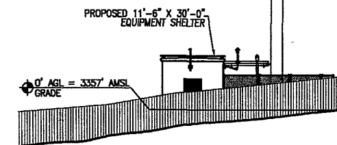
1 ELEVATION A-1 SCALE: 1/16"=1'-0"
