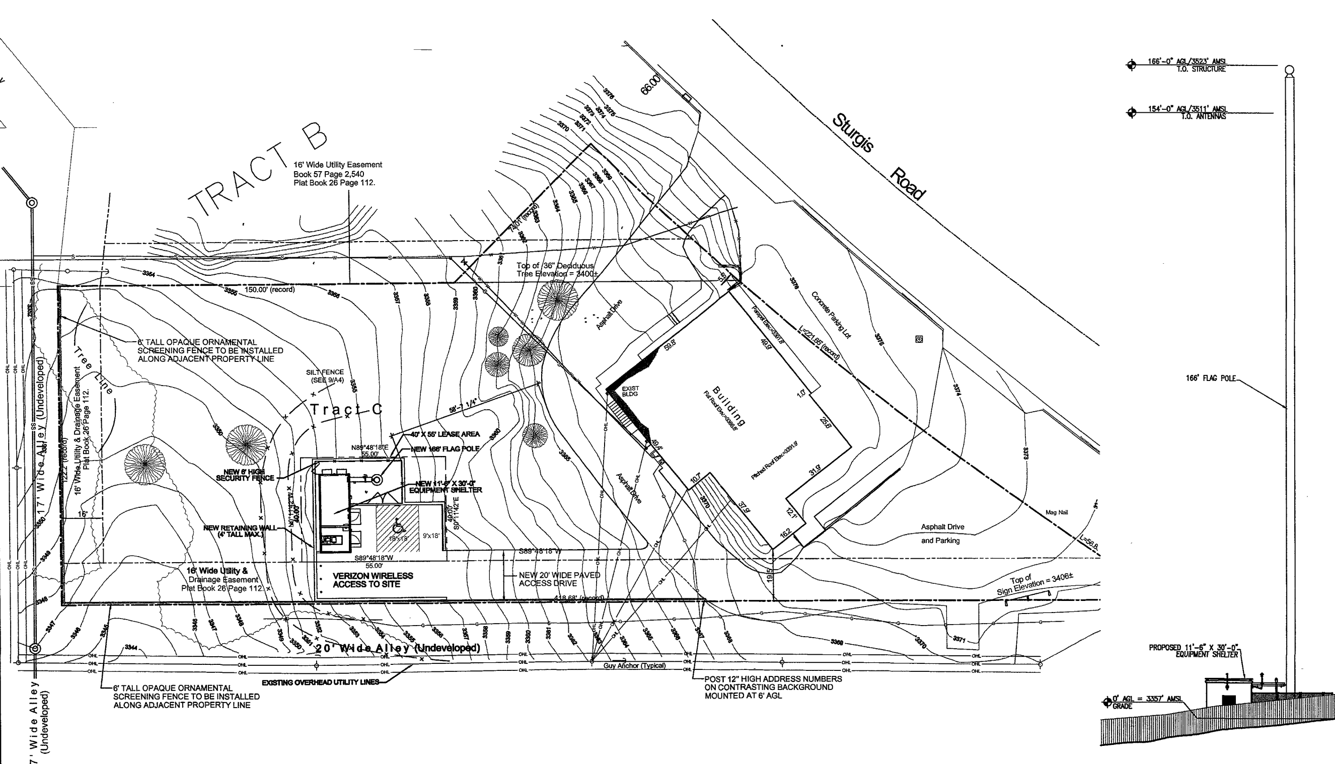
1 SITE PLAN A-1 SCALE: 1/16"=1'-0"
