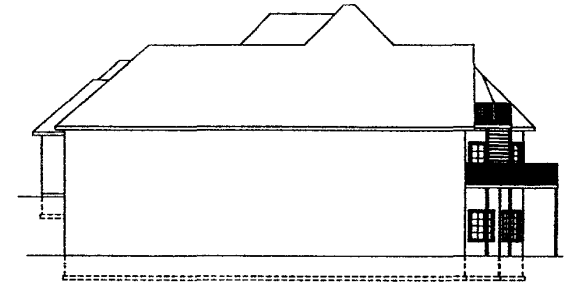
RIGHT ELEVATION
