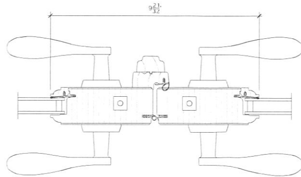
6 3 MEETING STILE SCALE: 6" = 1'-0"
