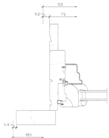
3 JAMB SCALE: 6" = 1'-0"
