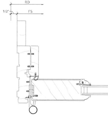
5 3 JAMB SCALE: 6" = 1'-0"
