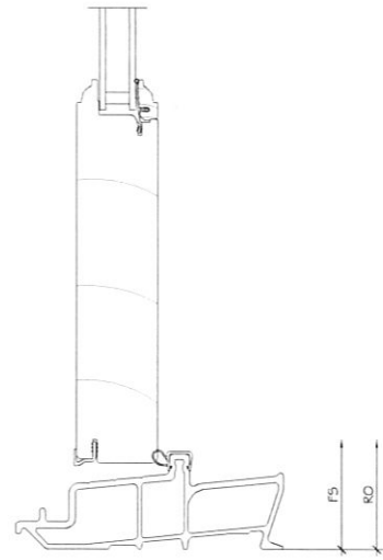
4 3 SILL SCALE: 6" = 1'-0"
