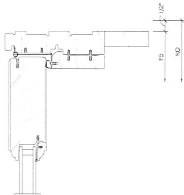
3 3 HEAD SCALE: 6" = 1'-0"
