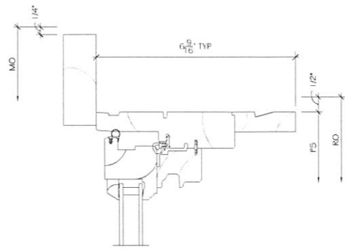
1 HEAD SCALE: 6" = 1'-0"
