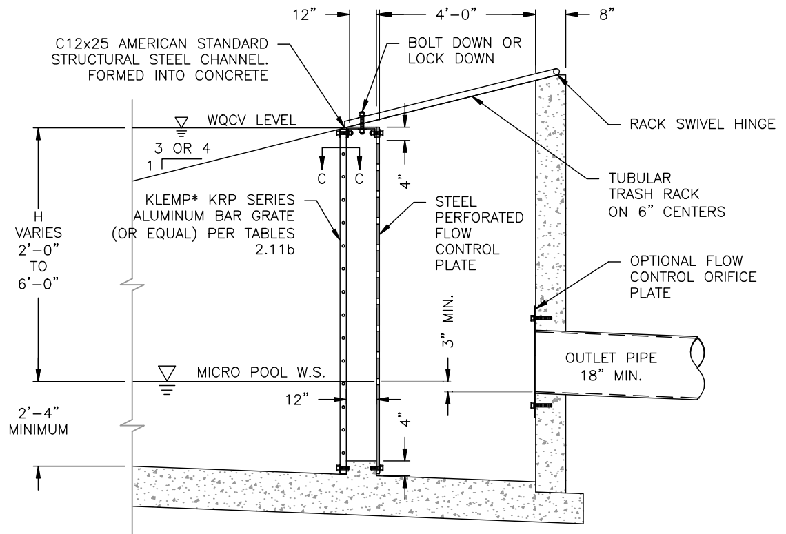
SECTION A-A
