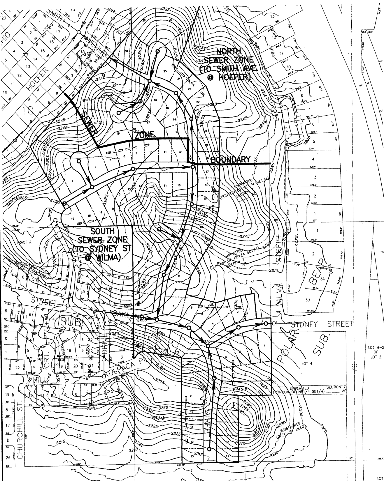
Park Meadows Subdivision Sewer Zone Plan
