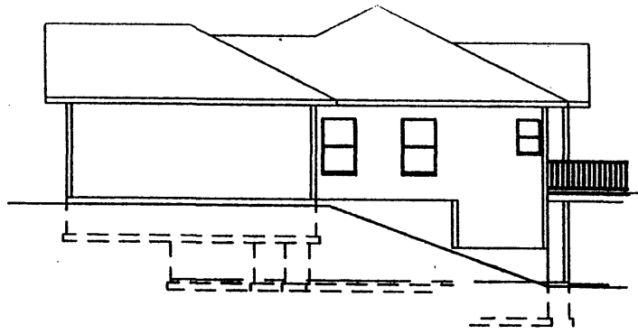
RIGHT ELEVATION
